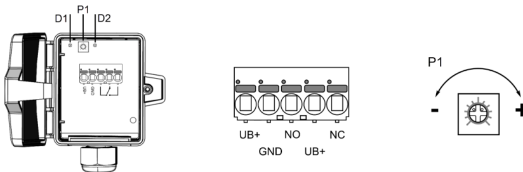
Abbildung 2: Montage SHX-9120
