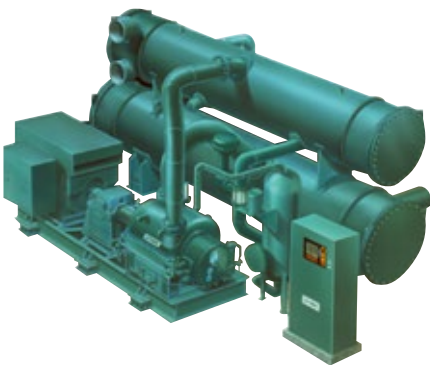
Titan OM HP Wasser-Wasser-WP Multi Turbotechnologie R1234ze Warmwasser bis zu 95°C Heizleistung: 5000 bis 20000kW
