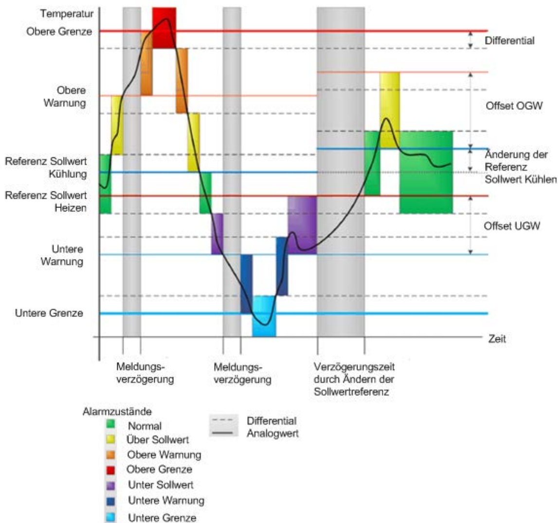
Abbildung 36: Heizung/Kühlung Sollwertmodus
