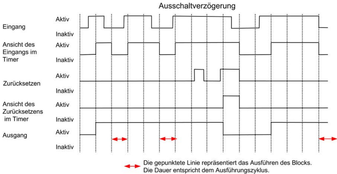
Abbildung 49: Ausschaltverzögerungstimer Beispiel 1
