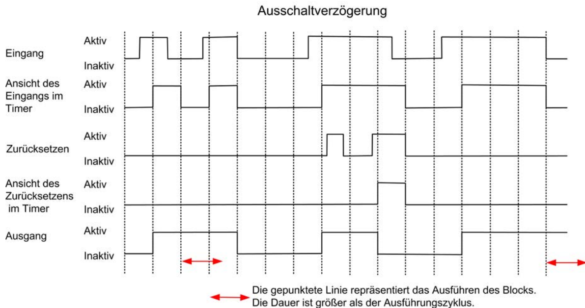
Abbildung 50: Ausschaltverzögerungstimer Beispiel 2
