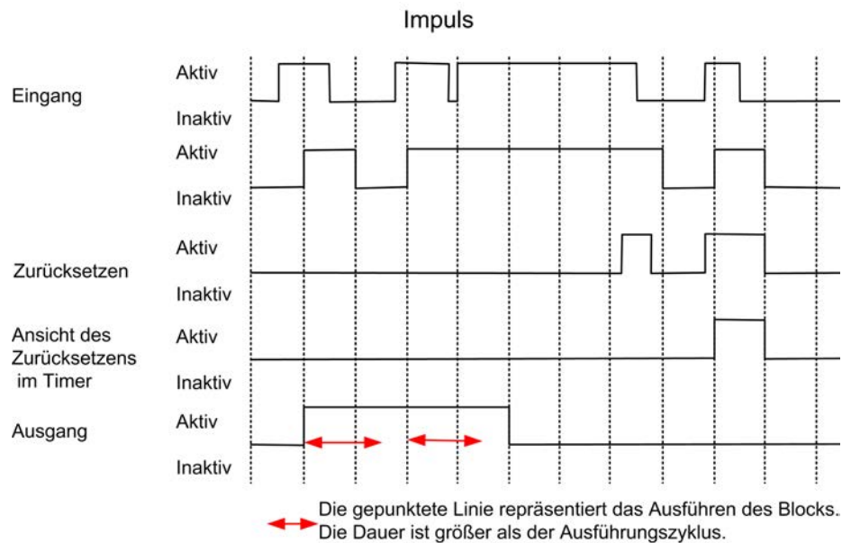
Abbildung 46: Impulstimer Beispiel 2
