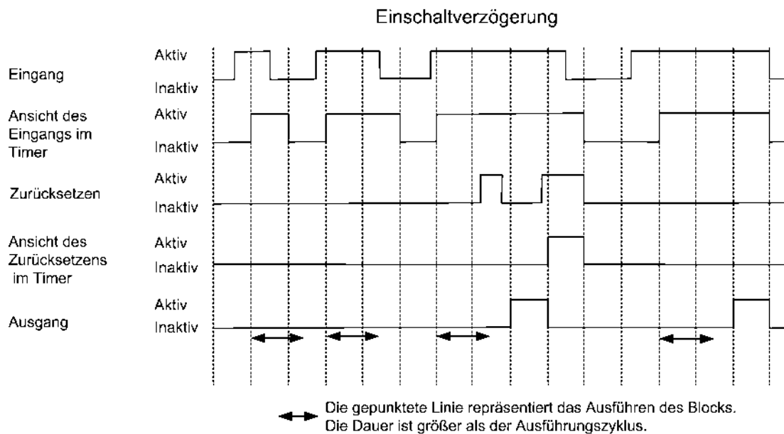
Abbildung 48: Timer Einschaltverzögerung Beispiel 2
