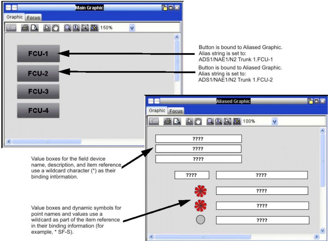
Abbildung 63: Beispiele für Alias-Hauptgrafik und Alias-Grafik
