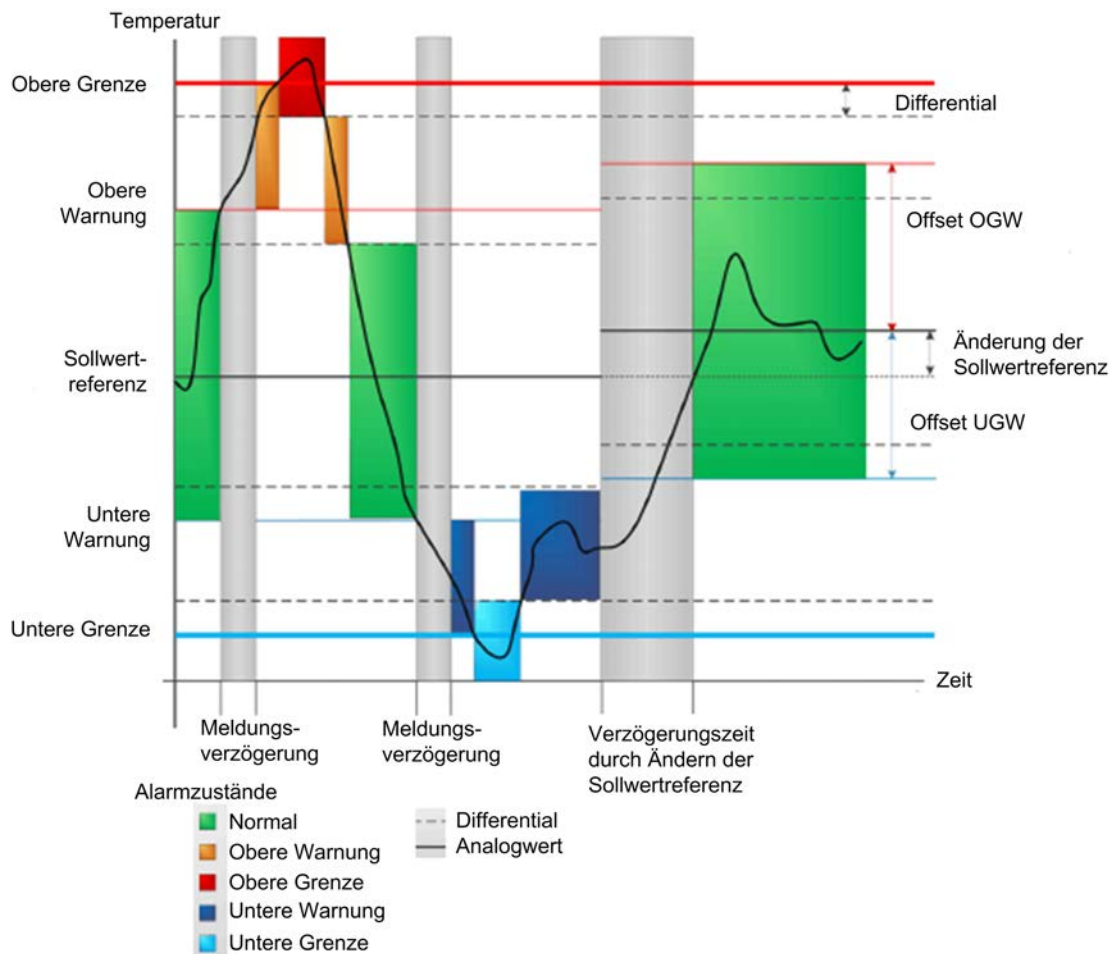
Abbildung 35: Modus Einzelsollwert
