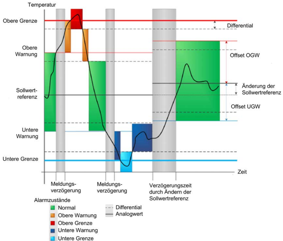
Abbildung 15: Modus Einzelsollwert
