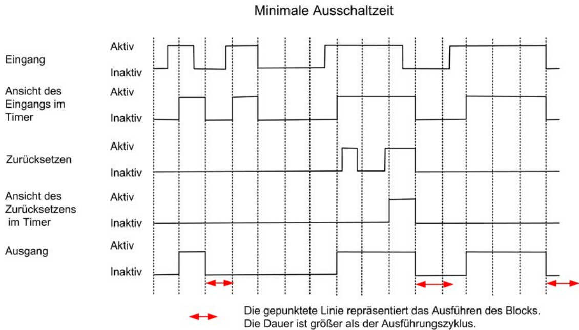
Abbildung 72: Timer für Min Ausschaltzeit Beispiel 2
