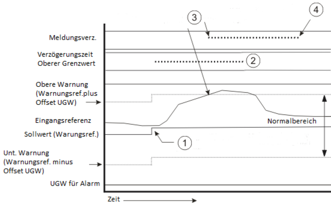
Abbildung 12: Zusammenspiel der verschiedenen Verzögerungszeiten
