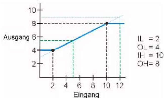
Abbildung 62: Funktionsbaustein Span Beispiel 2
