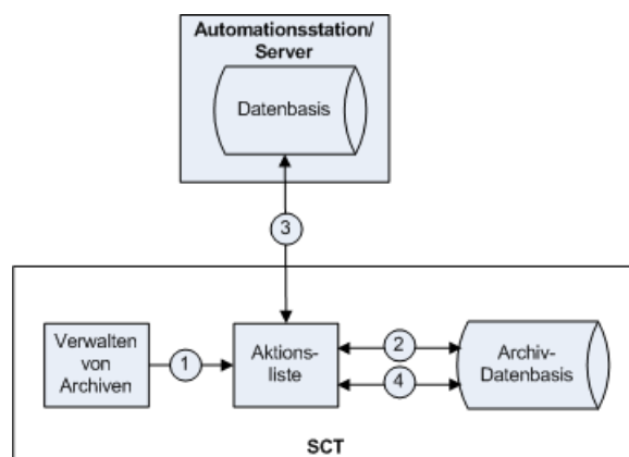
Abbildung 75: Synchronisierungsvorgang
