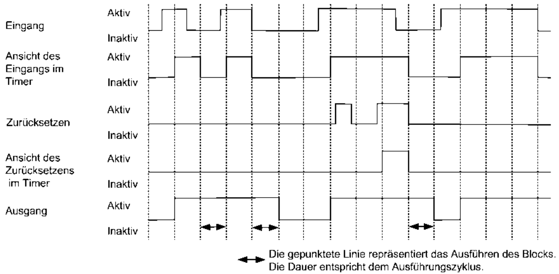
Abbildung 66: Timer Einschaltverzögerung Beispiel 2
