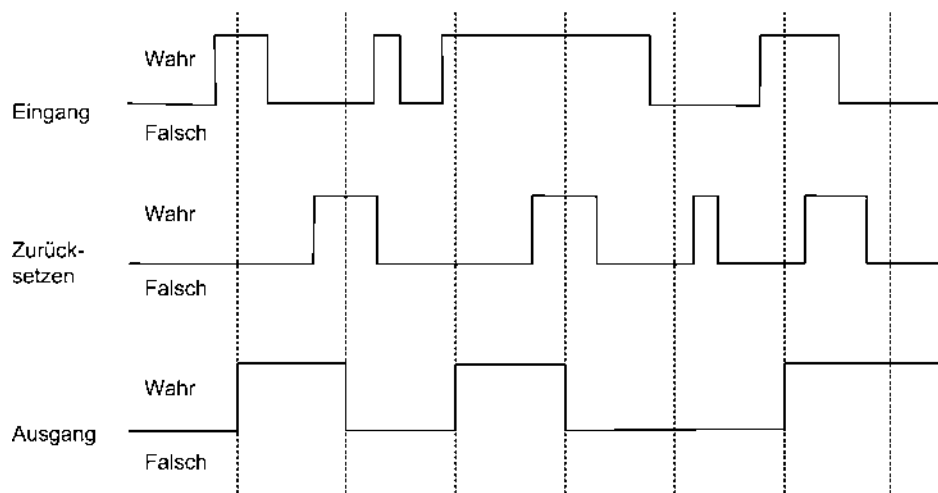
Abbildung 60: Beispiel für einen Funktionsbaustein vom Typ LTCH
