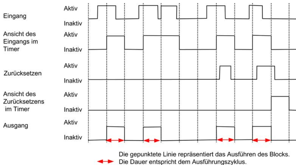
Abbildung 63: Impulstimer Beispiel 1
