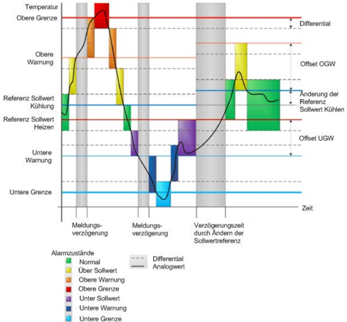
Abbildung 16: Heizung/Kühlung Sollwertmodus
