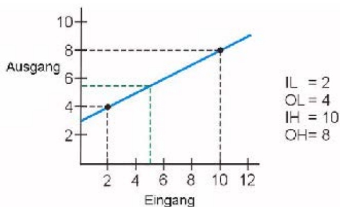
Abbildung 61: Funktionsbaustein Span Beispiel 1
