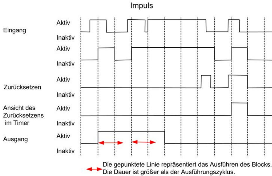
Abbildung 64: Impulstimer Beispiel 2
