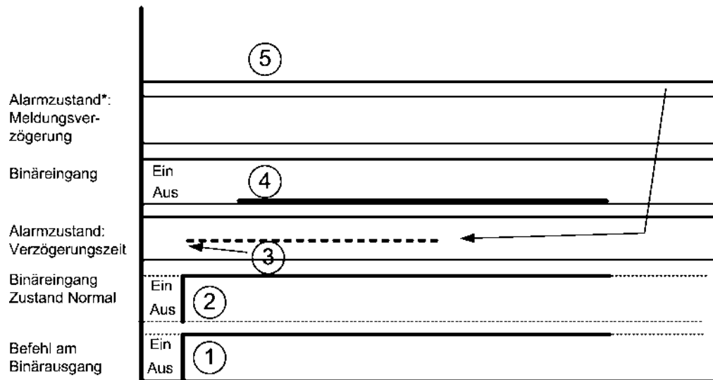
Abbildung 14: Ventilator hat einen Einschaltbefehl erhalten, funktioniert aber nicht
