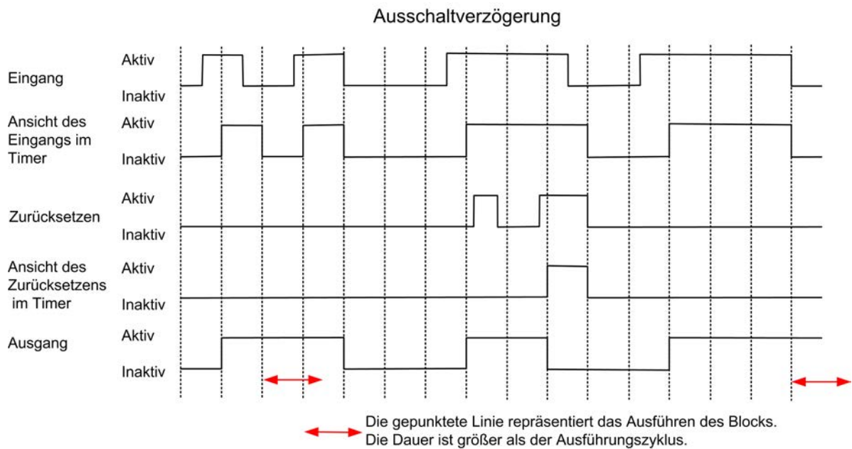
Abbildung 68: Ausschaltverzögerungstimer Beispiel 2
