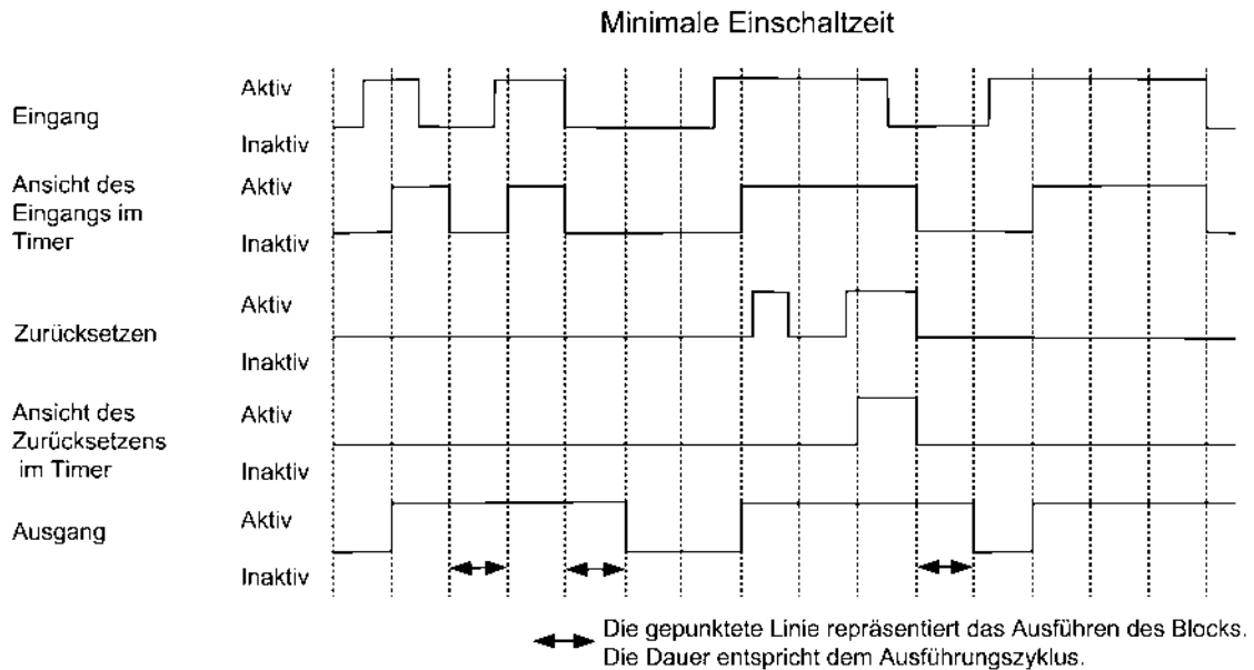
Abbildung 70: Timer für Min Einschaltzeit Beispiel 2
