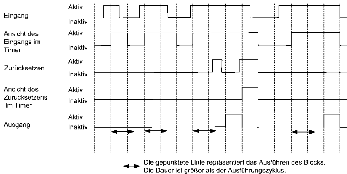
Abbildung 66: Timer Einschaltverzögerung Beispiel 2
