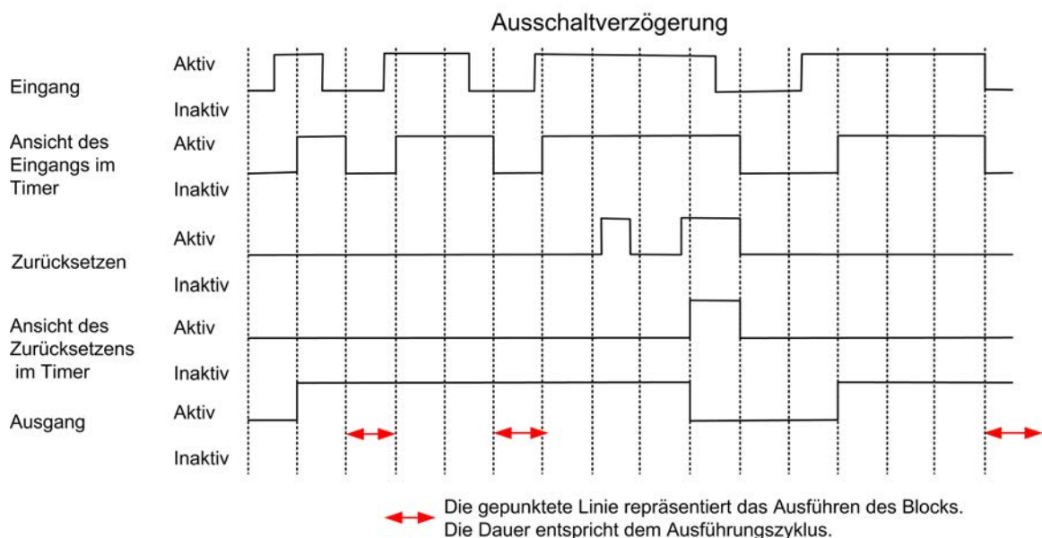
Abbildung 67: Ausschaltverzögerungstimer Beispiel 1
