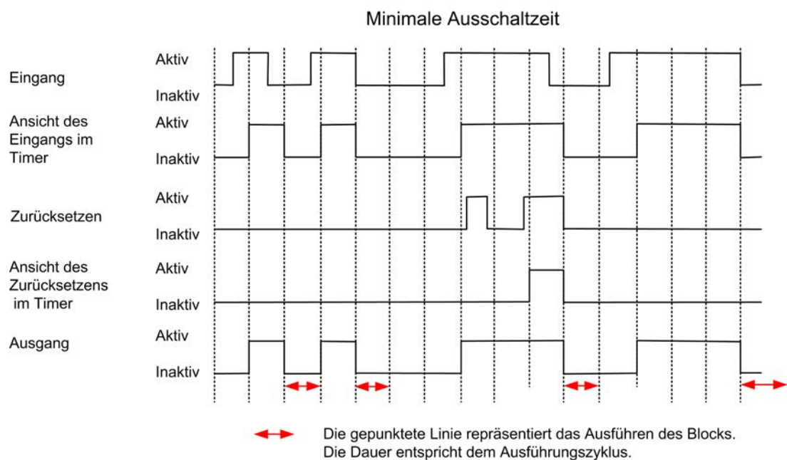
Abbildung 71: Timer für Min Ausschaltzeit Beispiel 1
