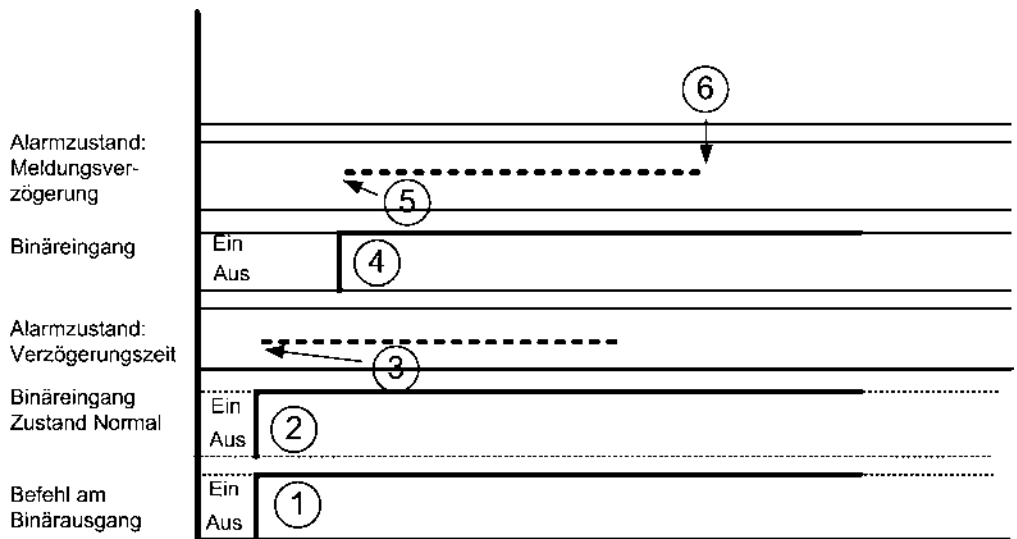
Abbildung 13: Ventilator ist eingeschaltet und läuft normal
