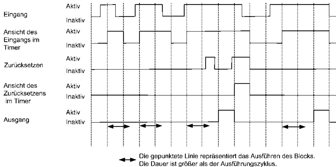
Abbildung 56: Timer Einschaltverzögerung Beispiel 2
