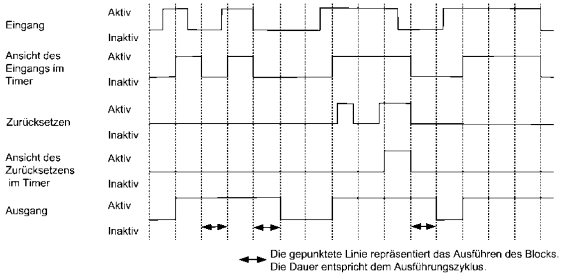
Abbildung 60: Timer für Min Einschaltzeit Beispiel 2
