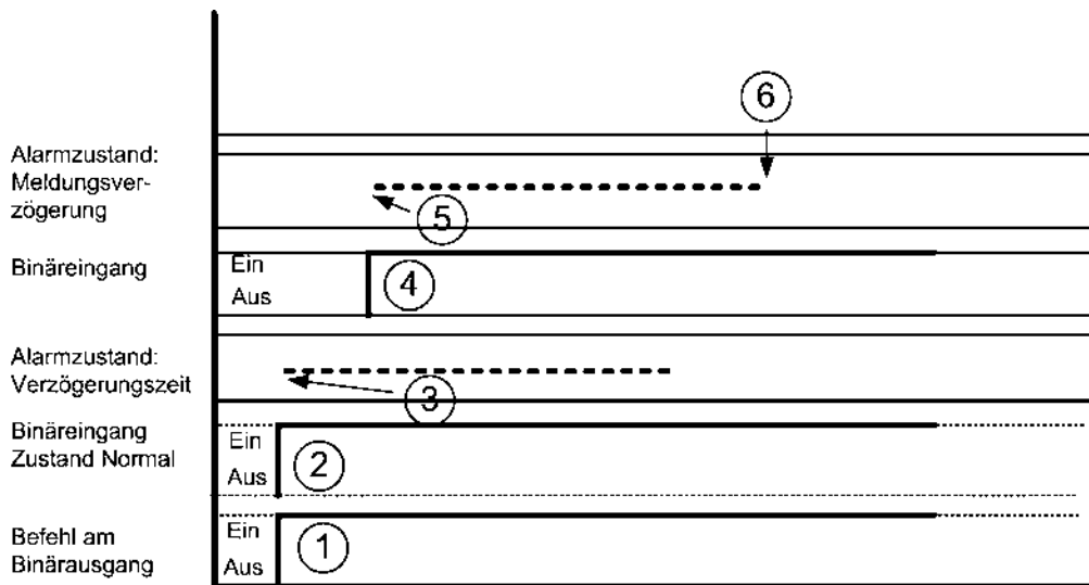
Abbildung 41: Ventilator ist eingeschaltet und läuft normal
