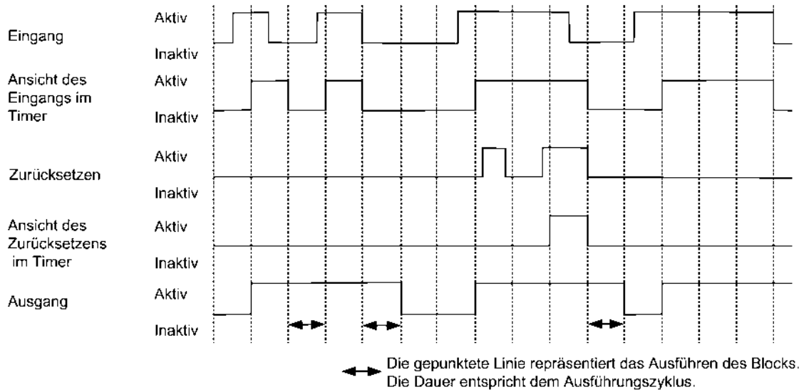
Abbildung 56: Timer Einschaltverzögerung Beispiel 2
